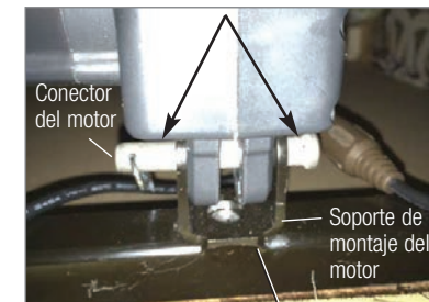
Las flechas muestran el conector del motor medianamente centrado en el soporte del motor
